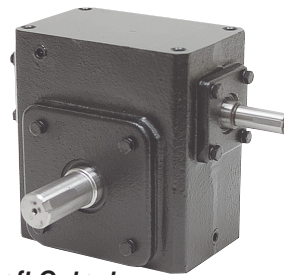
Left Output
