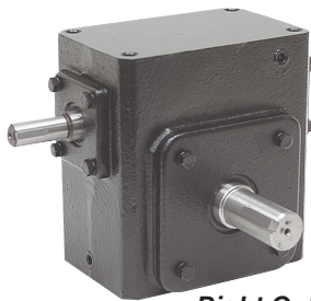
Right Output
